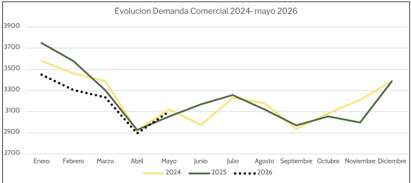
Figura 7: Evolución de la demanda de electricidad Residencial (GWh)
