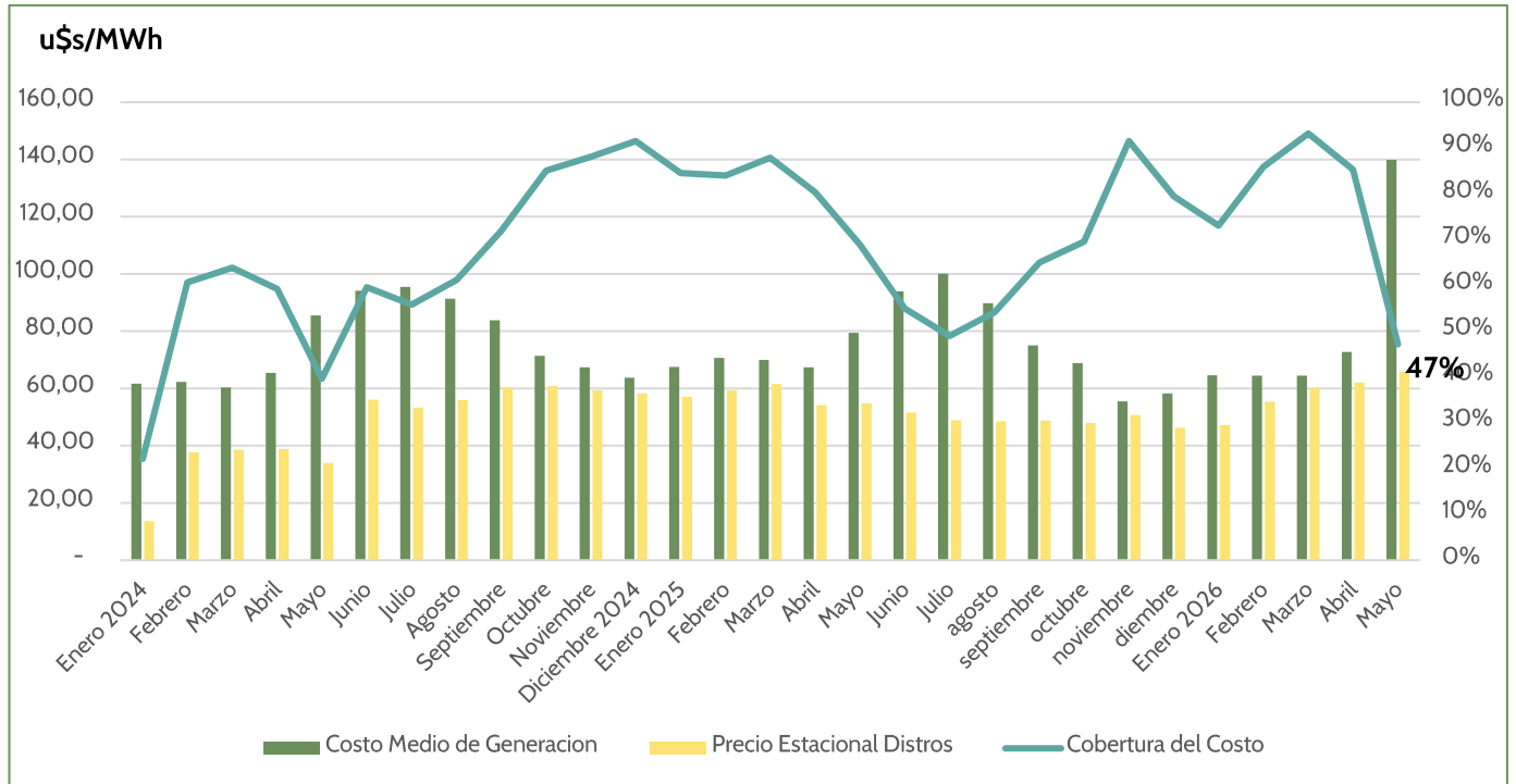
Figura 10: Evolución del costo medio de generación, precio mayorista Distribuidoras y cobertura de costos. 2024 - mayo 2026
