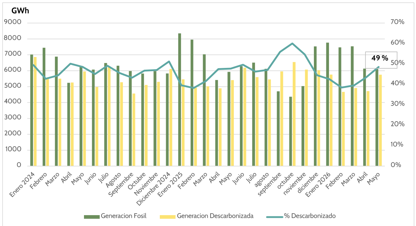
Figura 3: Generación fósil y descarbonizada (GWh), participación: 2024 - mayo 2026
